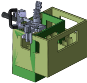
Hakentraverse für Saftkisten LHA 02.16A
