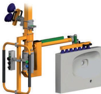
Vakuumtraverse für Waschbecken und Toilettenschüsseln mit Schnellwechselmechanismus für Traversenwechsel LVA 11.27A
