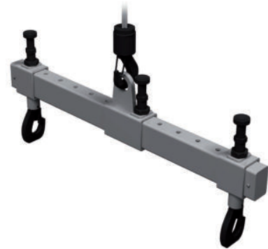
Manuell verstellbare Hakentraverser für Pumpen LHA 02.29A
