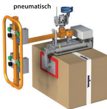
Parallelspanner für Kartons LPP 02.09A
