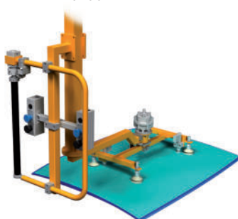
Vakuumtraverse mit 90° Drehantrieb für Glasscheiben LVA 14.04A
