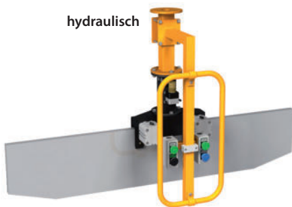
Schraubstockspanner für Flachstahl LPP 46.01A
