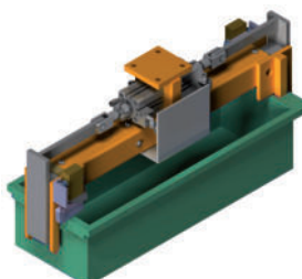
Parallelspanner KLT-Greifer für eine Größe Für zwei Größen mit manueller Schnellverstellung LPP 21.34A
