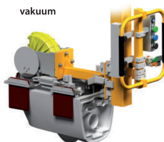
Spanner für WC-Rückwände LPP 33.27A
