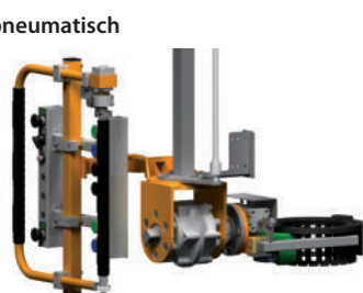
Parallelspanner mit Drehvorrichtung bis zu 270° für Statoren LPP 42.34A
