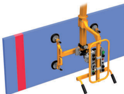
Vakuumtraverse inkl. 180° Drehantrieb für Kunststoffelemente oder/und Flachglas LVA 58.02A
