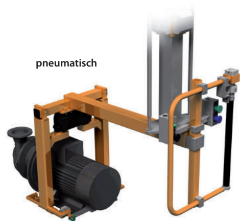
Parallelspanner für Pumpen LPP 03.28A
