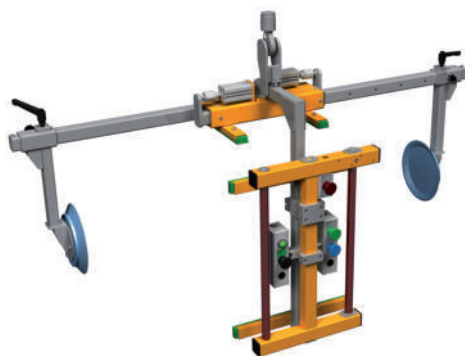
Pneumatisch verfahrbarer Vakuum- greifer für Büromöbel LVA 07.13A
