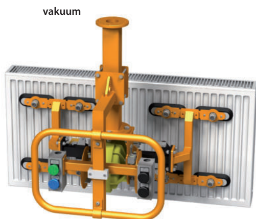
Vakuumtraverse inkl. 90° Schwenkantrieb für Heizkörper Konzeptbild
