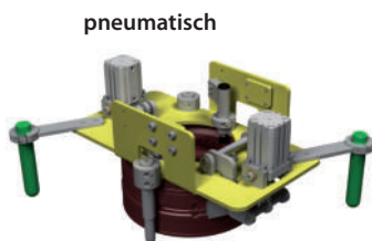
Parallelspanner für Statoren LPP 82.03A
