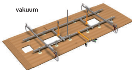
Vakuumtraverse für Wohnwagen Dach-, Seiten- und Bodenelemente LVA 69.02A
