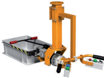
Gabelspanner mit 110° Drehantrieb für Stapelkisten LPP 54.02A
