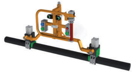
Scherenspanner für Wellen LSP 06.12A
