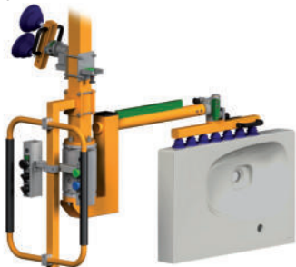
Vakuumtraverse für Waschbecken und Toilettenschüsseln mit Schnellwechselmechanismus für Traversenwechsel LVA 11.27A
