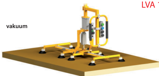
Vakuumtraverse mit 90° Schwenkvorrichtung für Duschwannen LVA 11.29A
