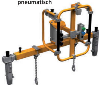
Parallelspanner für Linearführungen (Schneeberger) LPP 21.38A
