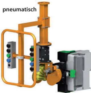
Parallelspanner inkl. 90° Schwenkantrieb für Wechselrichtergehäuse LPP 75.02A
