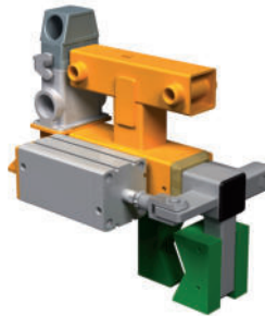
Parallelspanner für Wellen LPP 21.45A
