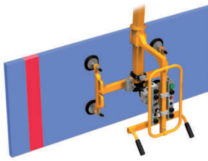
Vakuumtraverse inkl. 180° Drehantrieb für Kunststoffelemente oder/und Flachglas LVA 58.02A
