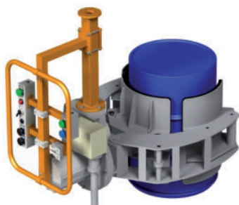
3-Backen-Spanner inkl. Drehvorrichtung für Fässer LPP 31.02A
