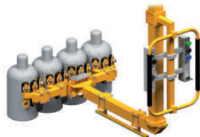
Vakuumtraverse mit Wechsel- Vorrichtung für verschiedene Saugereinheiten für (3 oder 4 Gasflaschen) LVA 20.21A
