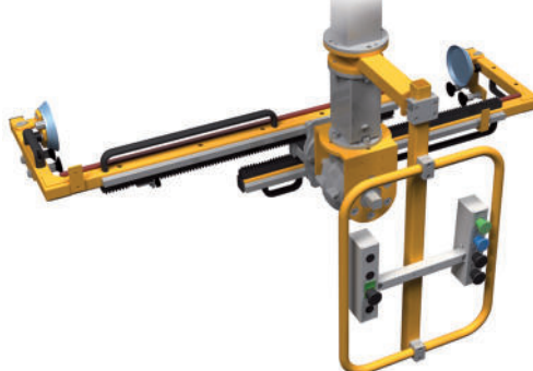
Manuell einstellbare Vakuumtraverse für Kühlschränke LVA 01.08A
