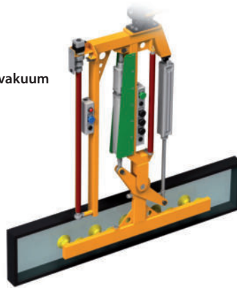
Vakuumtraverse inkl. 90° Schwenkvorrichtung für Glasscheiben LVA 62.01A
