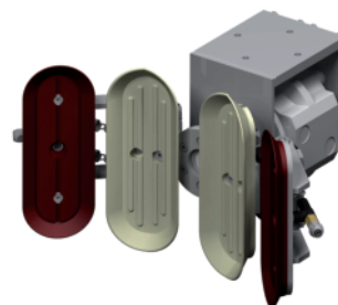
Vakuumgreifer mit 280° Drehvorrichtung für Boiler LVA 40.01A
