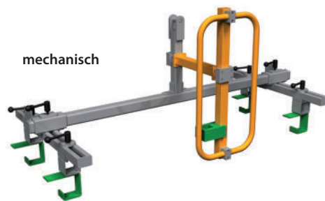
Manuell einstellbare Haken-traverse für Betten LHA 11.12A
