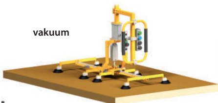
Vakuumtraverse für Waschbecken und Toilettenschüsseln mit Schnellwechselmechanismus für Traversenwechsel LVA 11.27A
