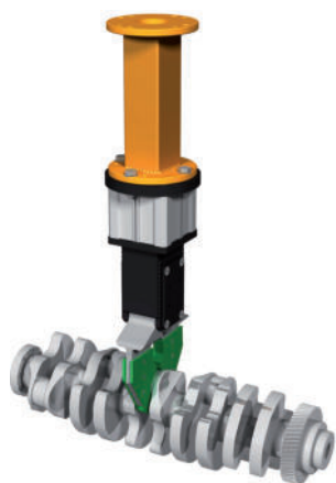
Scherengreifer für Kurbelwelle LSP 15.05A
