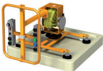
Vakuumtraverse inkl. 90° Schwenkantrieb für Duschtassen LVA 11.05A
