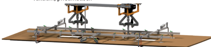
Vakuumtraverse mit pneumatisch betriebenen umklappbaren Haken zur Absturz-sicherung für Fußböden LVA 69.04A
