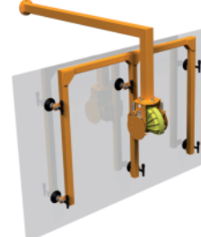
Vakuumtraverse mit 90° Schwenkvorrichtung für Glasscheiben LVA 10.13A
