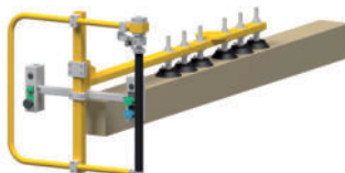
Vakuumtraverse für längliche Kartons LVA 01.10A
