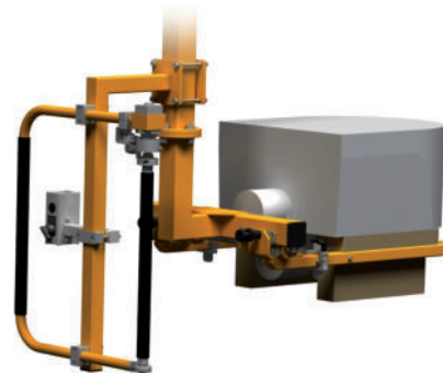
Gabelwerkzeug mit verstellbaren Greifbacken für verschiedene Toilettenschüsseln LHA 22.21A
