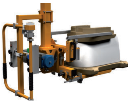
Parallelspanner mit verstellbaren Greifbacken und 180° Drehvorrich- tung für verschiedene Toiletten- schüsseln LHA 22.20A
