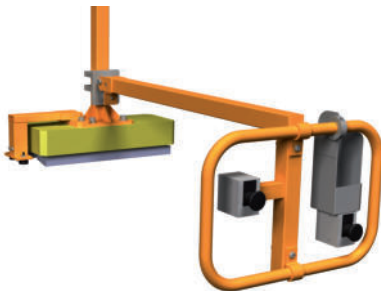
Magnettraverse für Luftkessel LMA 01.03A
