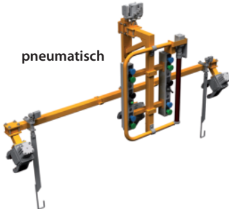
Scherenspanner mit einstellbarer Spann- position für Gelenkwellen LSP 06.18A
