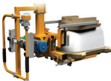
Parallelspanner mit verstellbaren Greifbacken und 180° Drehvorrichtung für verschiedene Toiletten- schüsseln LHA 22.20A
