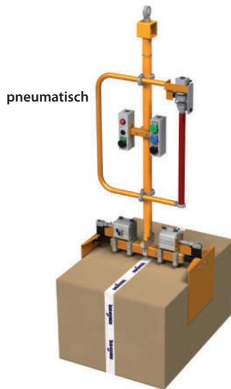
Parallelspanner für Kartons LPP 02.10A
