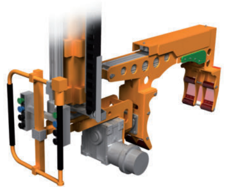
Parallelspanner für Druckluftkessel LPP 62.03A
