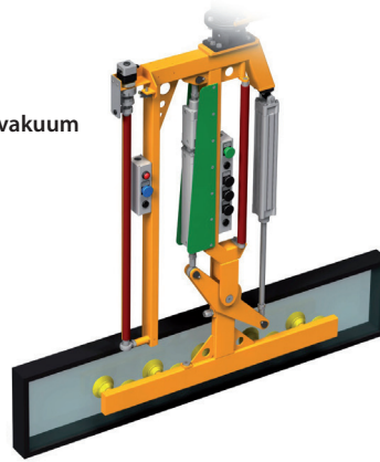
Vakuumtraverse inkl. 90° Schwenkvorrichtung für Glasscheiben LAM - Nr. LVA 6201
