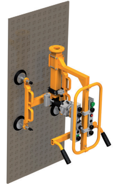
Vakuumtraverse inkl. 90° Schwenkantrieb für Glasscheiben LAM - Nr. LVA 3801
