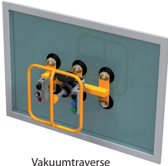
Vakuumtraverse inkl. 180° Drehvorrichtung für Fenster LAM - Nr. LVA 1011
