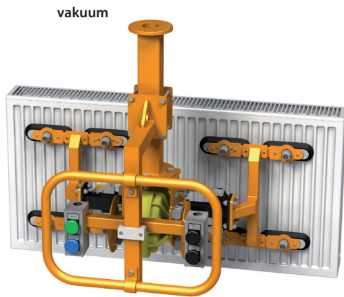
Vakuumtraverse inkl. 90° Schwenkantrieb für Heizkörper
