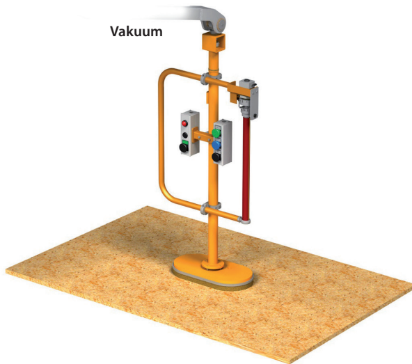
Vakuum-Flächensauger für Spanplatten
