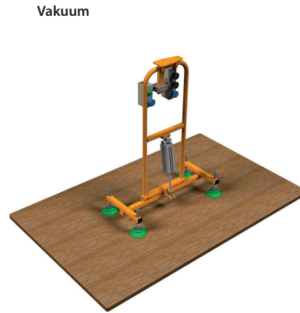
Vakuumtraverse mit 90° pneumatischer Schwenkvorrichtung für Holzplatten LAM - Nr. LVA 0705
