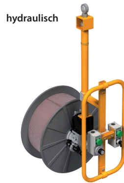
3 Backengreifer für Drahtspulen LAM - Nr. LPP 3803
