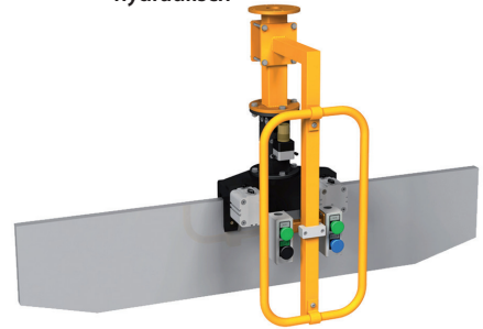
Schraubstockspanner für Flachstahl LAM - Nr. LPP 4601
