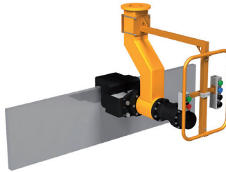
Schraubstockspanner inkl. 180° Drehantrieb für Flachstahl LAM - Nr. LPH 0802
