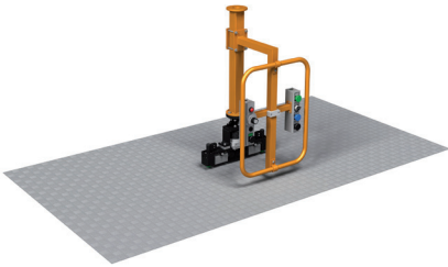
Magnettraverse für Bleche LAM - Nr. LMA 0101
