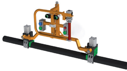
Scherenspanner für Wellen LAM - Nr. LSP 0612
