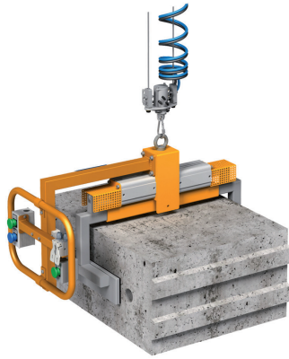
Parallelspanner für Gasbetonelemente LAM - Nr. LPP 5701
