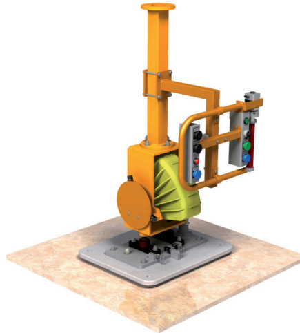
Vakuum-Flächenspanner mit 90° Schwenkantrieb für Fliesen LAM - Nr. LVA 0703
