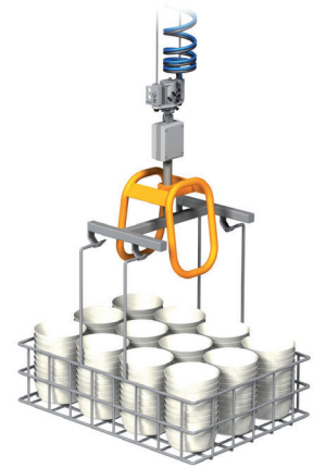
Hakentraverse mit Waage für Transportkörbe LAM - A.-Nr. 2251
