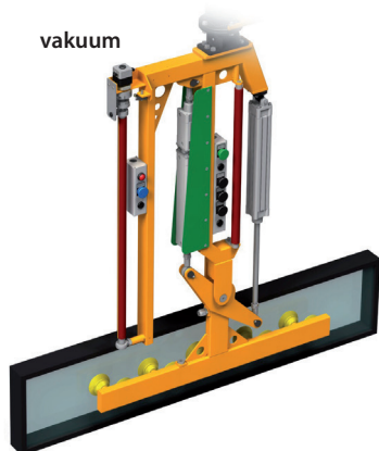
Vakuumtraverse inkl. 90° Schwenkvorrichtung für Glasscheiben LAM - Nr. LVA 6201
