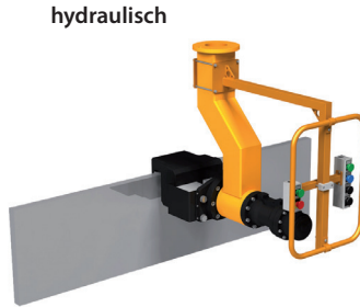
Schraubstockspanner inkl. 180° Drehtrieb für Flachstahl LAM - Nr. LPH 0802
