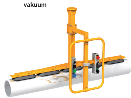
Vakuumgreifer für Rohre LAM - Nr. LVA 5901
